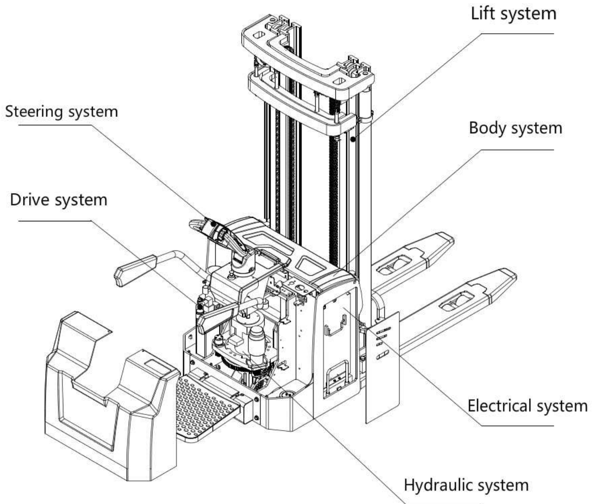
Сборка штабелера
