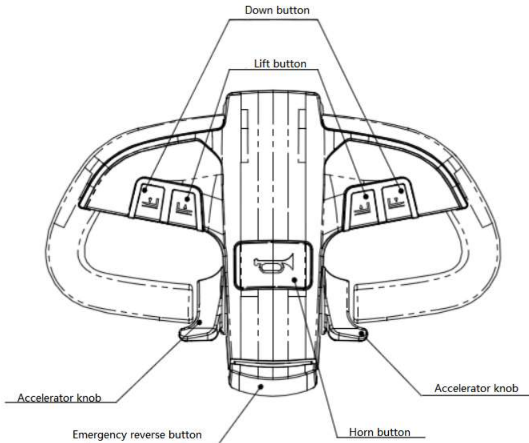
Ручка управления
